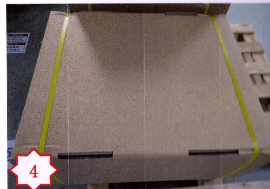
图四，确认 PA3236 无漏装后，将 32 的内箱与外箱配合后，并打包装带待出货。
